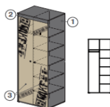
Шкаф 814x598x2164
