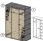
Шкаф-окончание 598x402x2164
